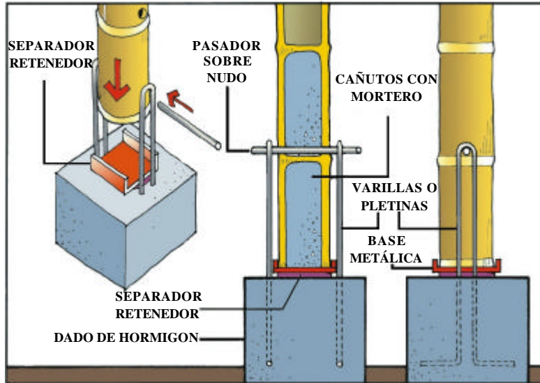
Figura E-B.2.1 Conexión cemento – columna de guadua con separador en pletina
