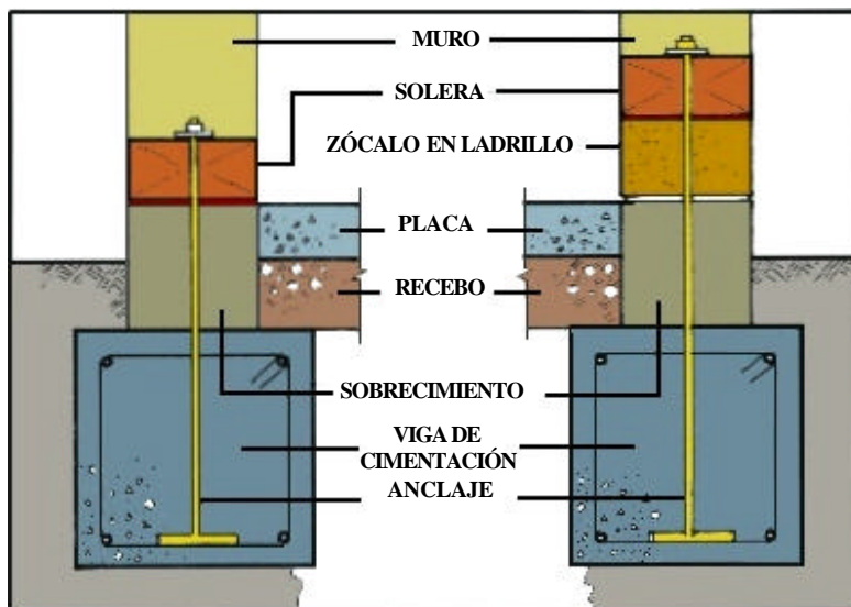
Figura E-B.2 Conexión cemento – columna de guadua con separador tubular
