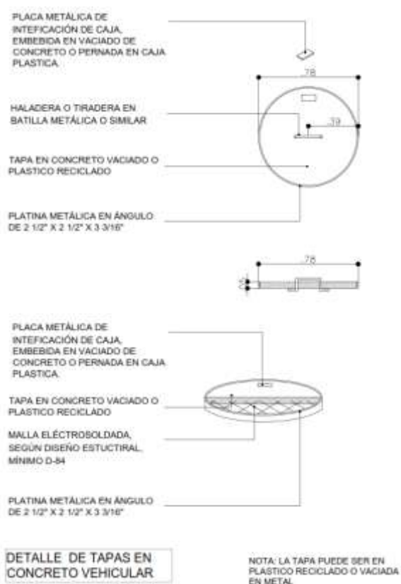
Gráfica 8. Detalle de construcción de la tapa circular
