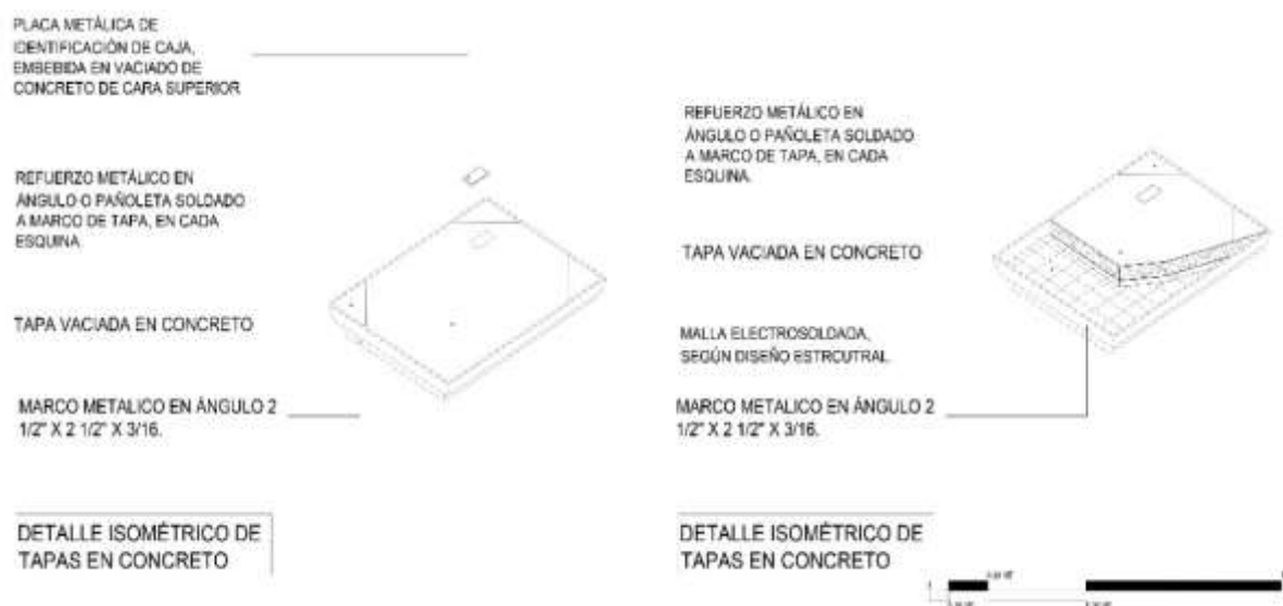
Gráfica 7. Detalle de construcción de la tapa
