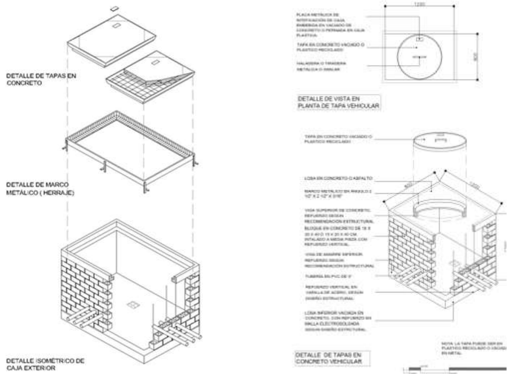
Gráfica 4. Composición cámara de entrada y enlace
