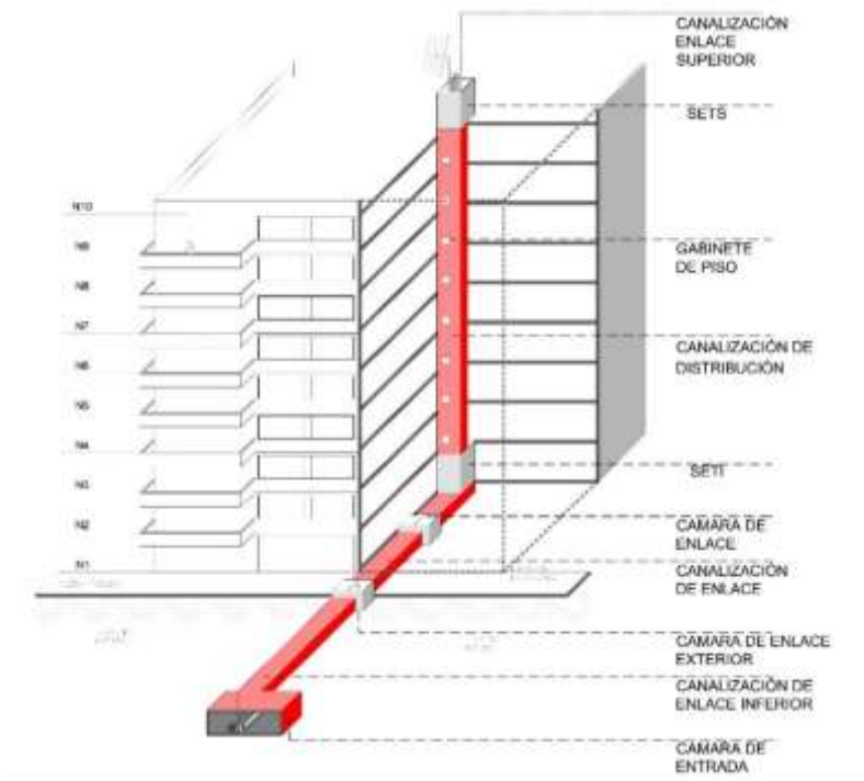
Gráfica 3. Infraestructura Soporte
