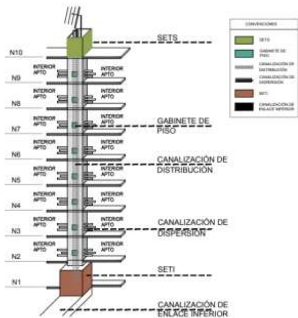
Gráfica 10. Esquema de canalización de distribución en edificios de varios pisos
