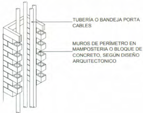
Gráfica 9. Detalle del Buitrón
