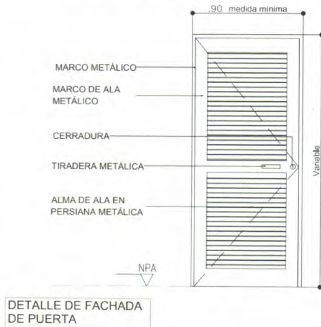
Gráfica 7. Detalle de la puerta
