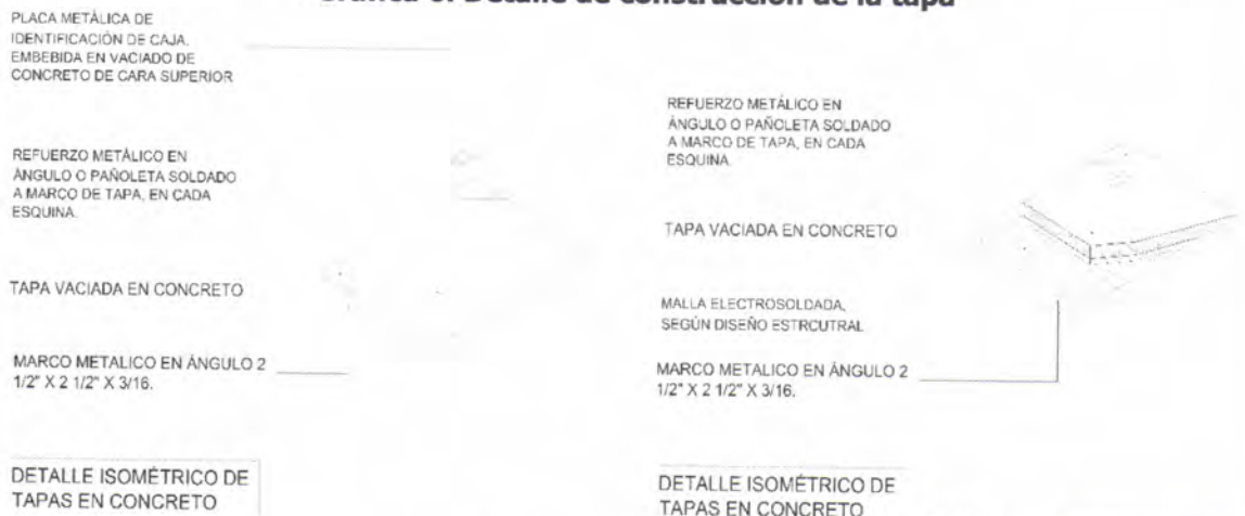
Gráfica 6. Detalle de construcción de la tapa
